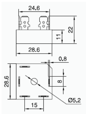
外形图:
